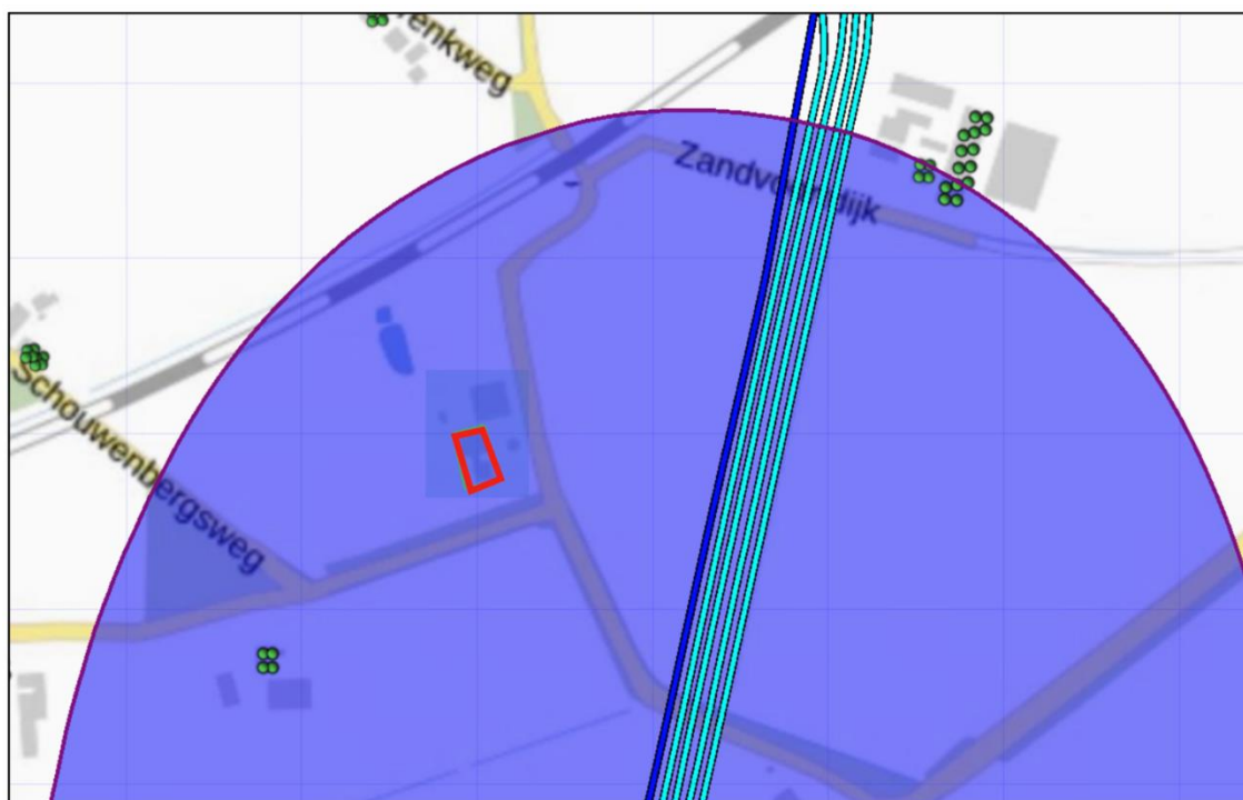
Figuur 3.1 Plaatsgebonden risico voor 7305_leiding-A-662-deel-1 van N.V. Nederlandse Gasunie
