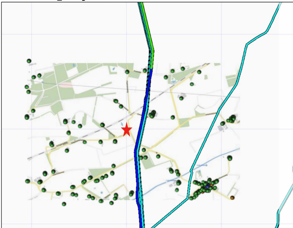
Figuur 4.2 Kilometer leiding behorende bij de maximale overschrijding van de FN-curve voor 7305_leiding-A-662-deel-1 van N.V. Nederlandse Gasunie
