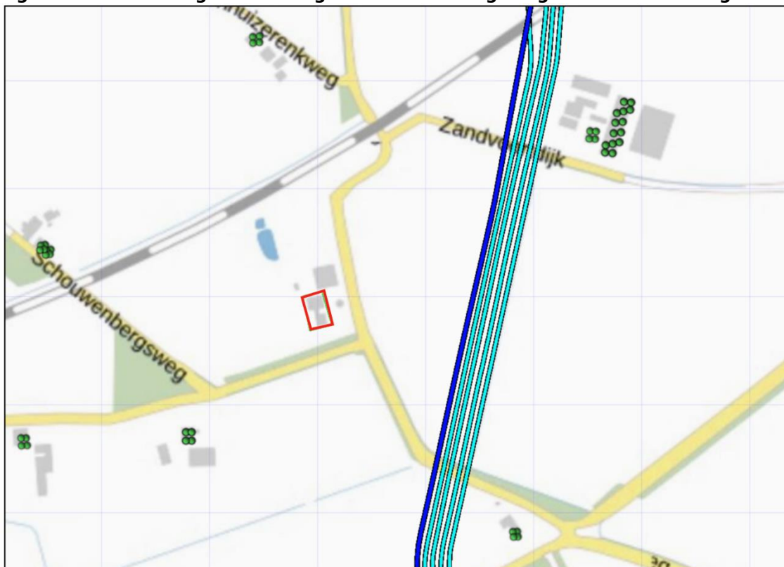
Figuur 2.2 Buisleidingen aanwezig in de directe omgeving van het interessegebied
