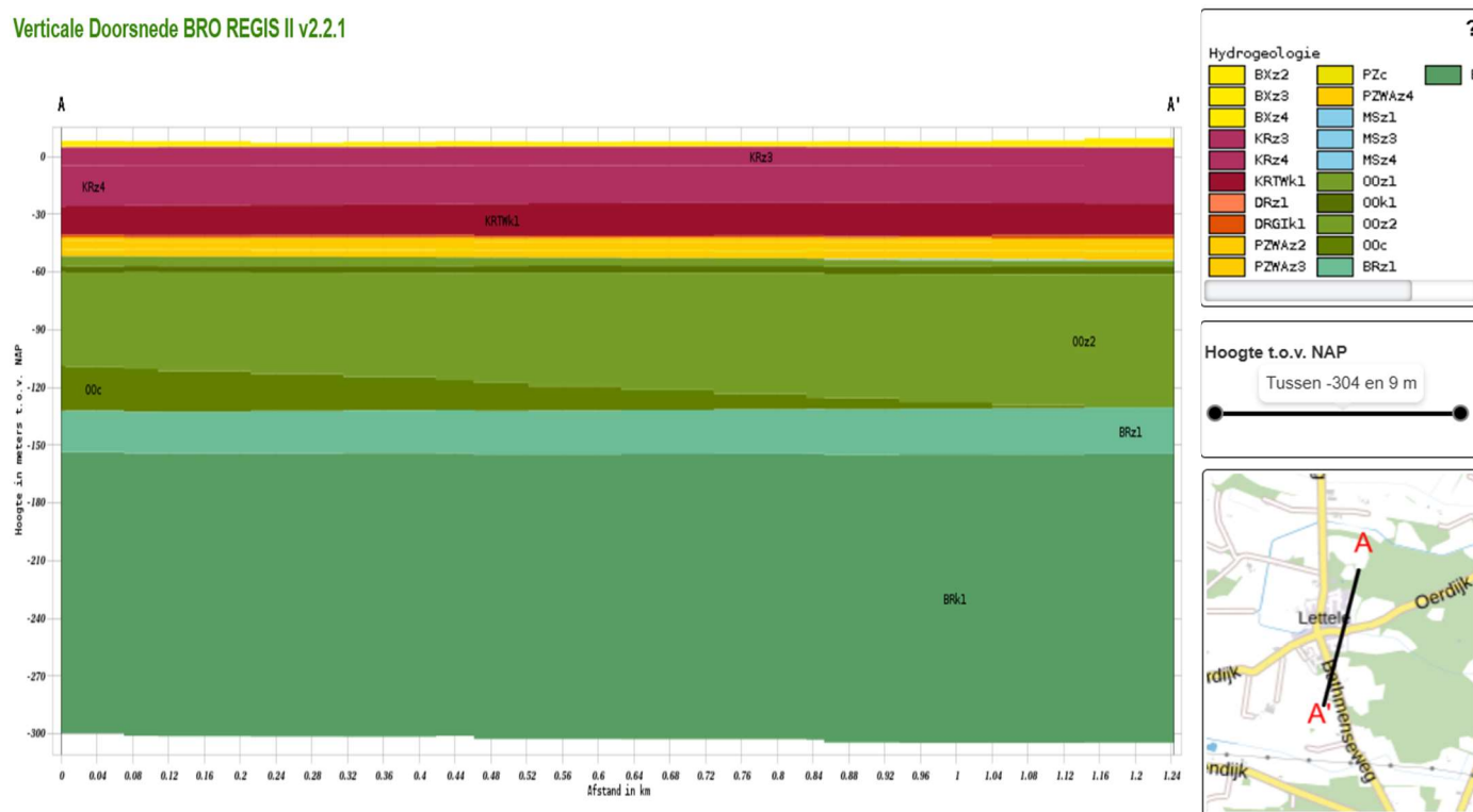
Figuur 3: De geohydrologische opbouw
